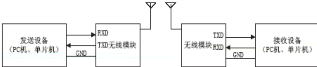
图（二）无线传输应用框图
