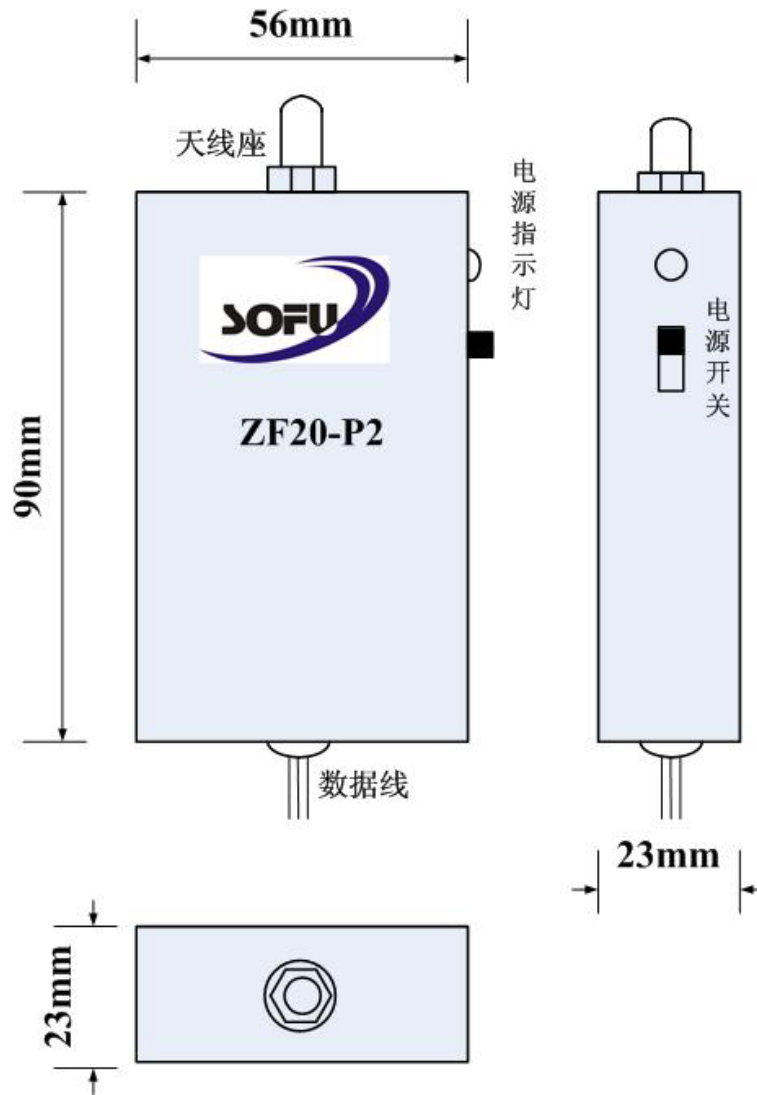
图（一）接口与尺寸
