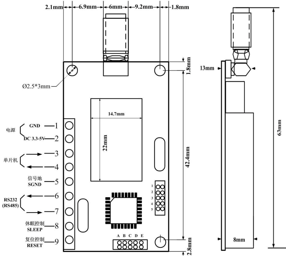
图（一）接口与尺寸
